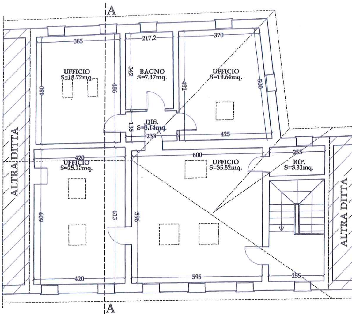
PIANTA PIANO SECONDO 1:100 REALIZZATO
